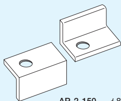
AP-2-150 φ8.0~φ21.5
