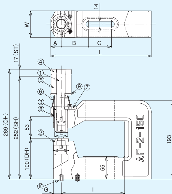
AP-2-150 φ8.0~φ21.5
